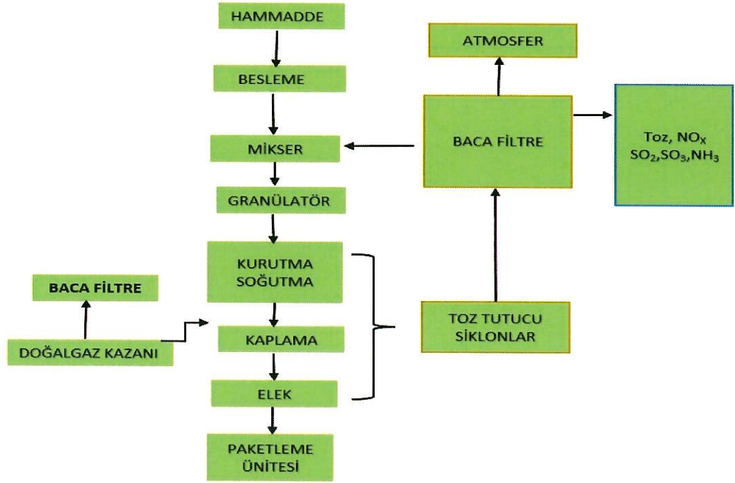
Samsun Granül GÜbre Üretim Tesisi İş Akımı Şeması
